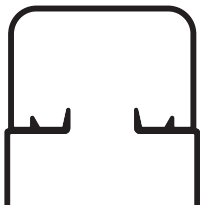
MA - 3034 Cabezal cubrebañera Peso: 0,767 kg/m
