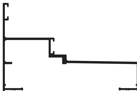
AH - 211 Jamba / umbral ventiluz Peso: 0,640 kg/m
