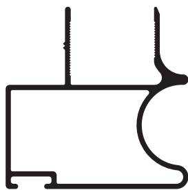
FP - 3401 Frente placard Peso: 0,418 kg/m
