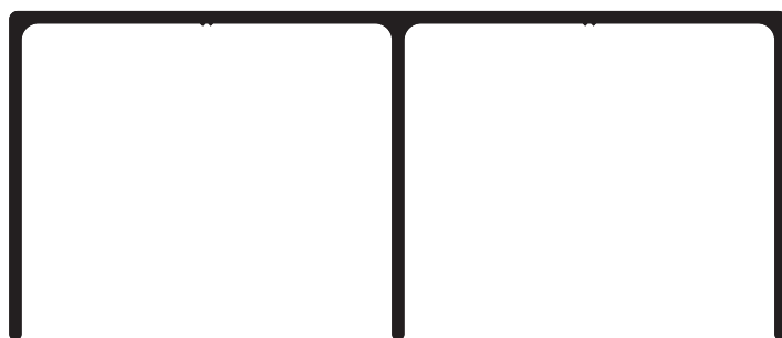
FP - 3402 Guía superior placard Peso: 0,845 kg/m
